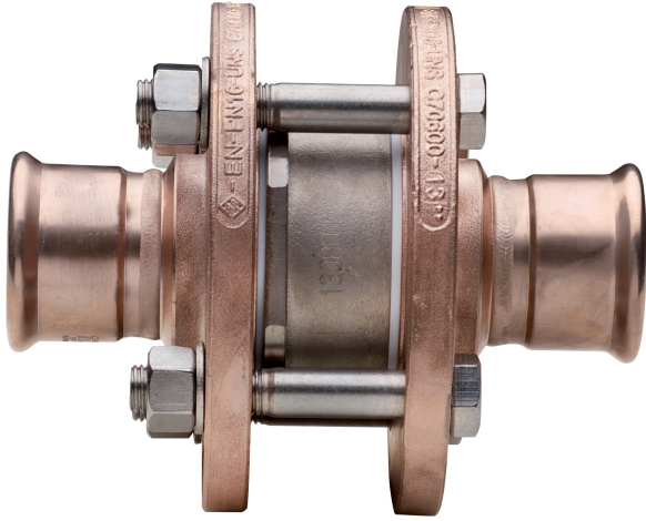
Disco-Rückschlagventil PN16.
